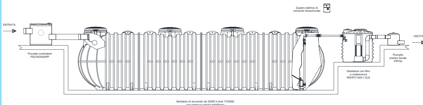
Figura 1: Sistema per il trattamento in accumulo delle acque di prima pioggia (ITIPP5000DOFC).
