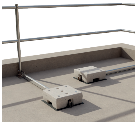
Versione 1 - con veletta \geq 15 cm
