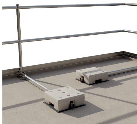
Versione 2 - con veletta \geq 5 cm < 15 cm
